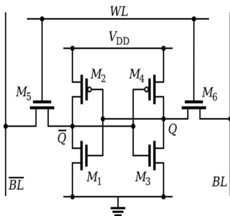
Fig.1 6T SRAM
