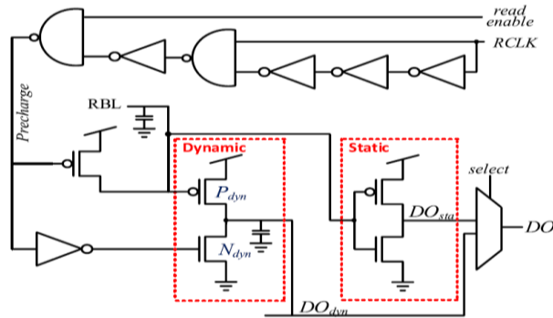
Fig.4. ReadOut Circuitry
